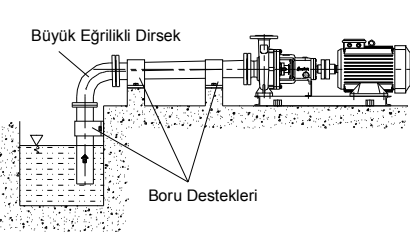
Şekil 5a. Emme Derinlikli
