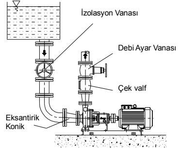
Şekil 6b. Emme Yükseklikli
