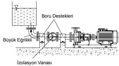
Şekil 5b. Emme Yükseklikli
