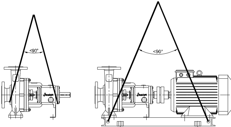
Şekil 1a. Çıplak Pompa
