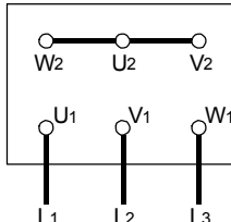
Şekil 13b. Y – bağlantı
