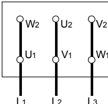
Şekil 13a. \Delta - bağlantı
