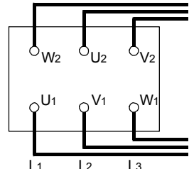
Şekil 13c. Y / \Delta - bağlantı
