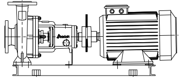
Şekil 4b. Düşey düzlemde açısal hata ve düzeltilmesi
